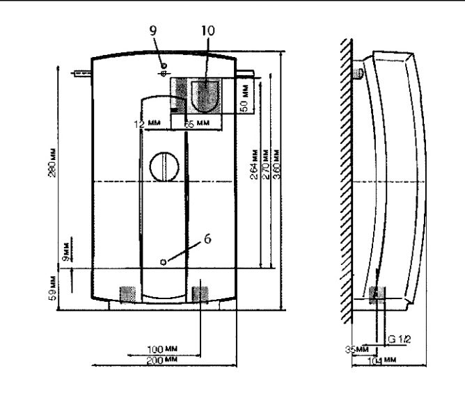
Расположение прибора
